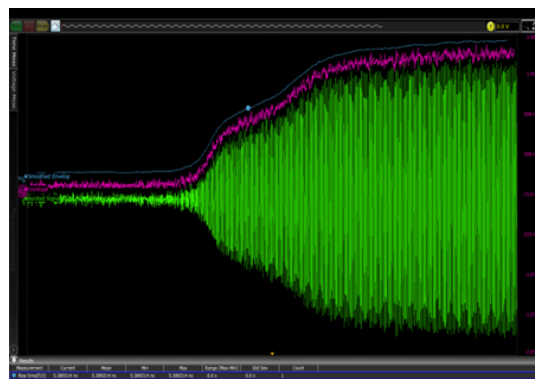
Амплитудная демодуляция.
